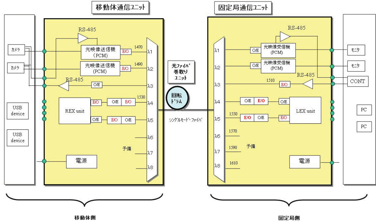
提案 構成図
